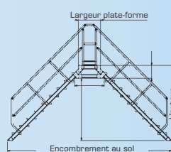
Inclinaison 45°
