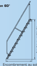
Inclinaison 60°
