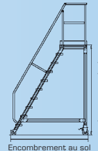
Inclinaison 60°
