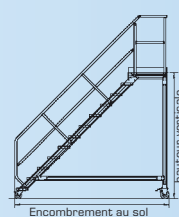
Inclinaison 45°
