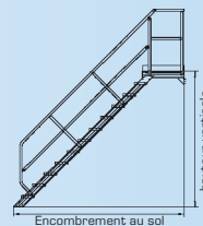
Inclinaison 45°
